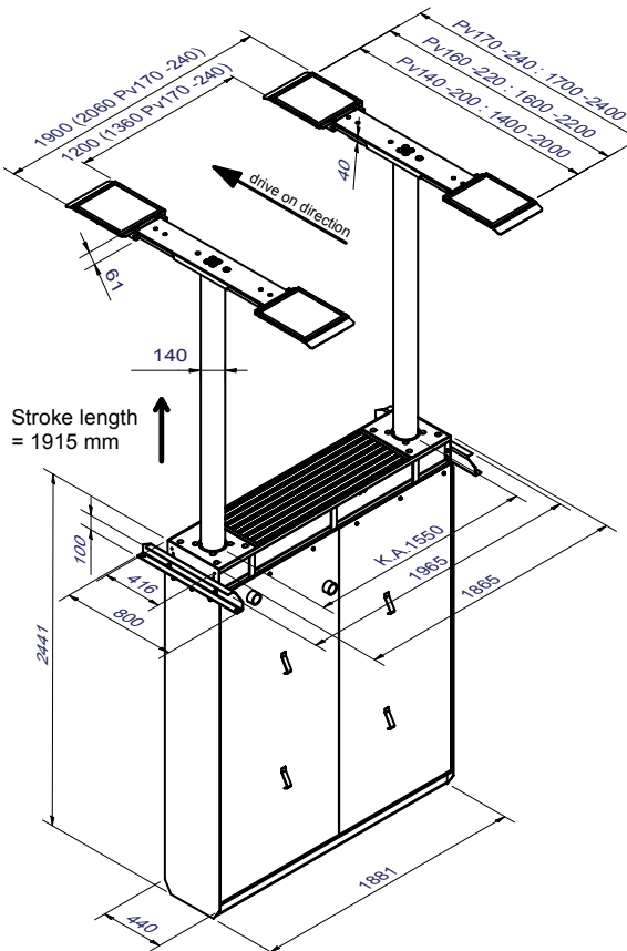
Supporti XY realizzati in una speciale lega di alluminio XY-pads available are made of a special aluminium alloy
